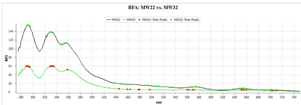
Figura 1: BFA - Esempio di buona corrispondenza tra le curve di due piezometri, attestante la probabile connessione idraulica tra di essi
