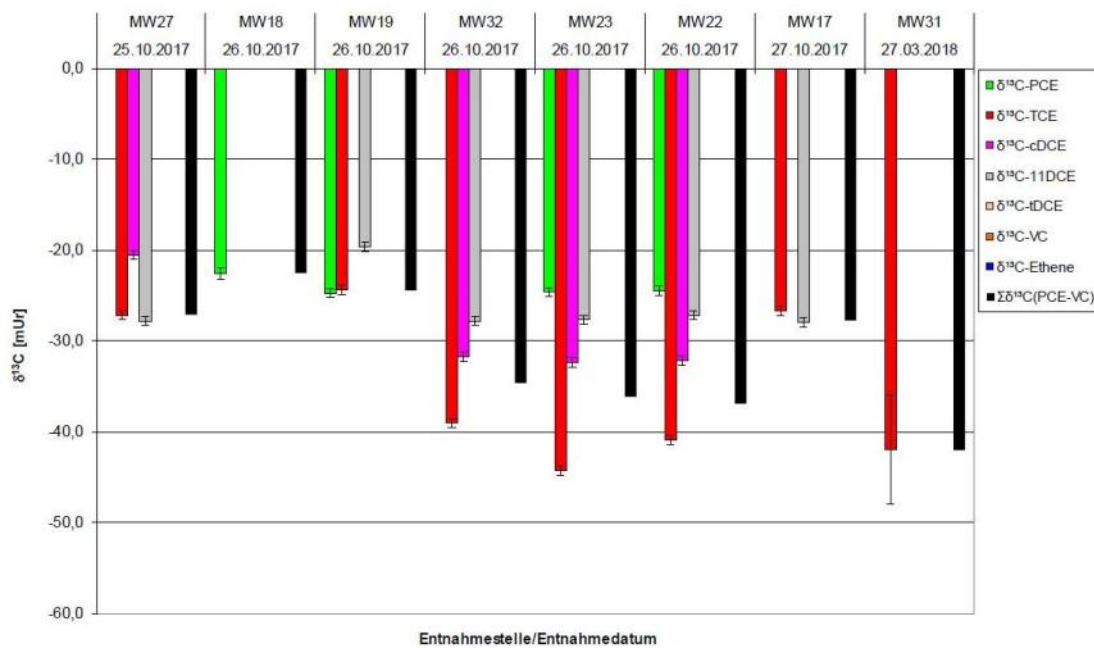
Figura 2: CSIA - Valori di \delta^{13}C ottenuti nelle stazioni di campionamento
