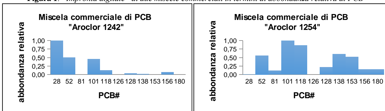
Figura 1. "Impronta digitale" di due miscele commerciali in termini di abbondanza relativa di PCB
