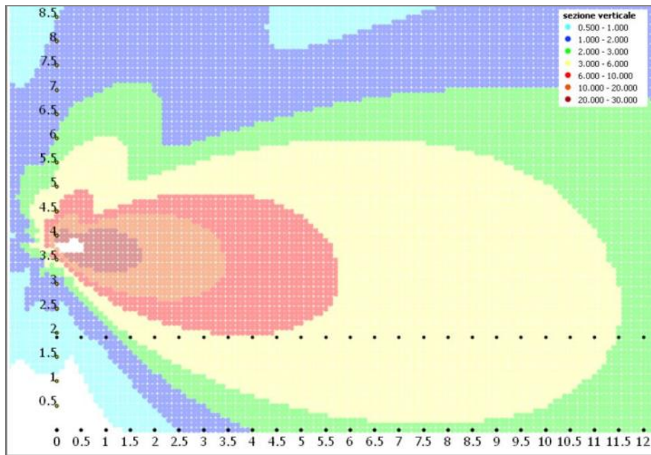
Figura 2 - Distribuzione del campo elettrico calcolato intorno ad una microcella per telefonia
