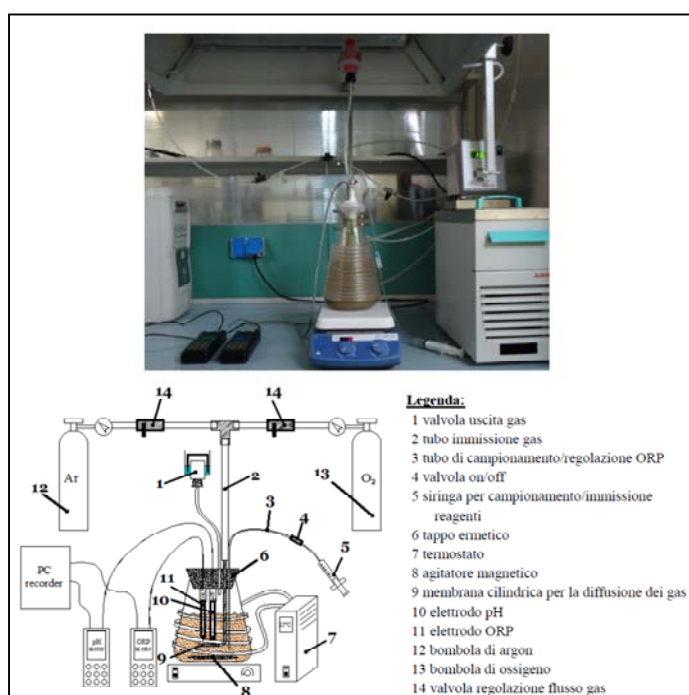
Figura 1: Apparato utilizzato durante le prove sperimentali di rilascio di arsenico: foto e schema.
