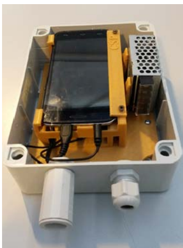
Postazione di monitoraggio a basso costo contenente lo smartphone
