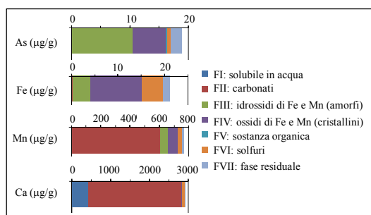
Figura 2: Partizionamento di As, Fe, Mn e Ca nella matrice solida dell'acquifero ottenuto tramite estrazioni selettive sequenziali
