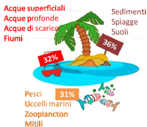
Figura 2. Distribuzione delle microplastiche nell'ambiente: dati derivanti da 170 articoli scientifici pubblicati.
