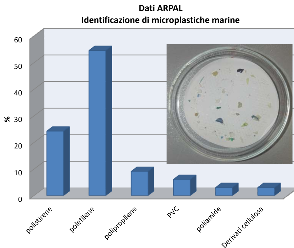
Figura 1. Distribuzione percentuale di plastiche e microplastiche presenti nei mari italiani
